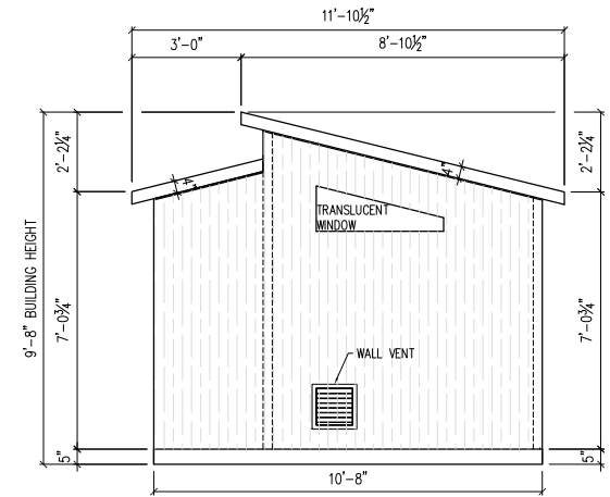
RIGHT ELEVATION
