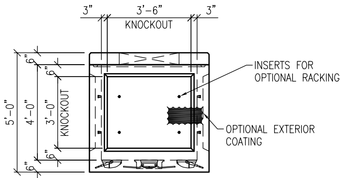
VIEW A SCALE: 1/4" = 1'-0"
