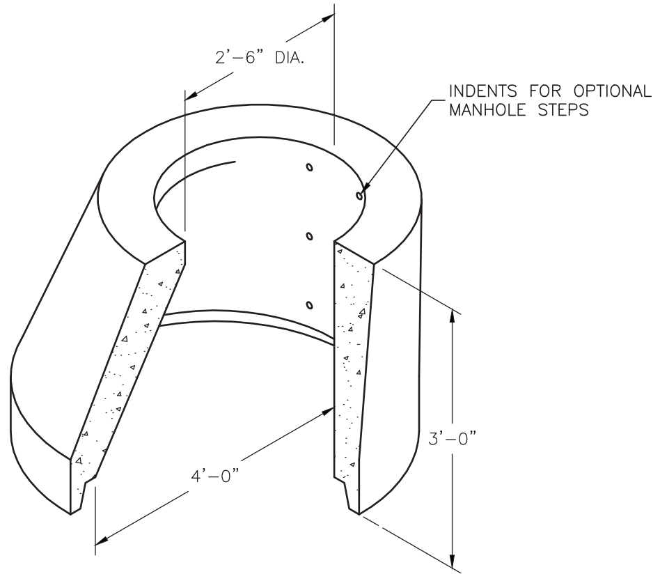
48" X 30" MANHOLE ECCENTRIC CONE
