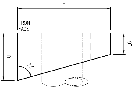
VIEW B SCALE: 1/2" = 1'-0"
