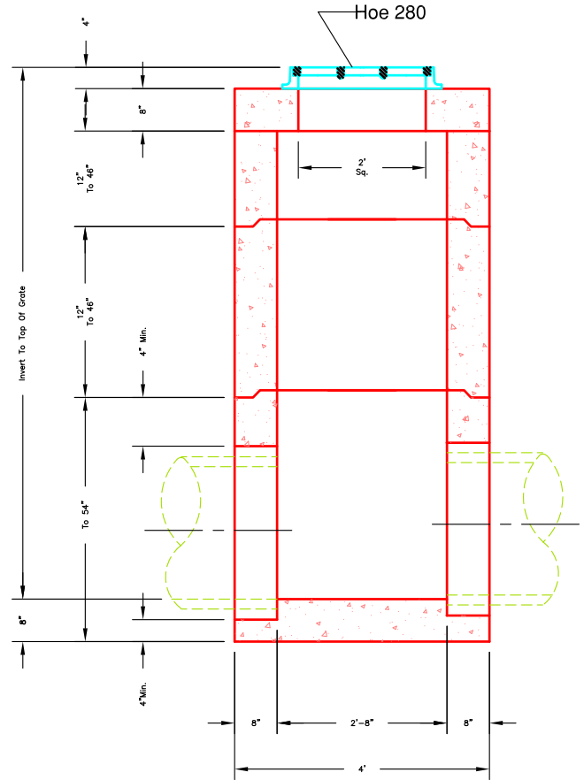
SECTION A-A
