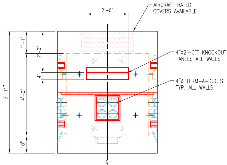
SIDE VIEW SCALE: 3/8" = 1'-0"
