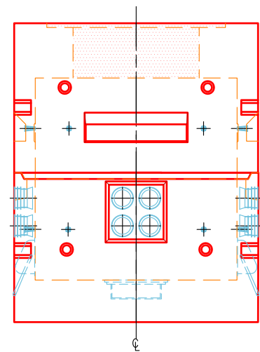
END VIEW SCALE: 3/8" = 1'-0"
