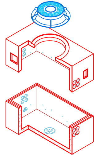
ISO VIEW SCALE: 1/8" = 1'-0"
