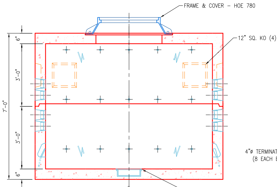
SIDE VIEW SCALE: 3/8" = 1'-0"
