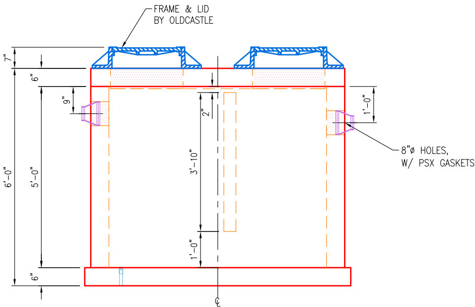
SIDE VIEW SCALE: 3/8" = 1'-0"
