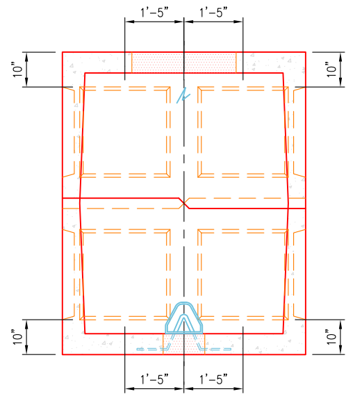
END VIEW SCALE: 5/16" = 1'-0"
