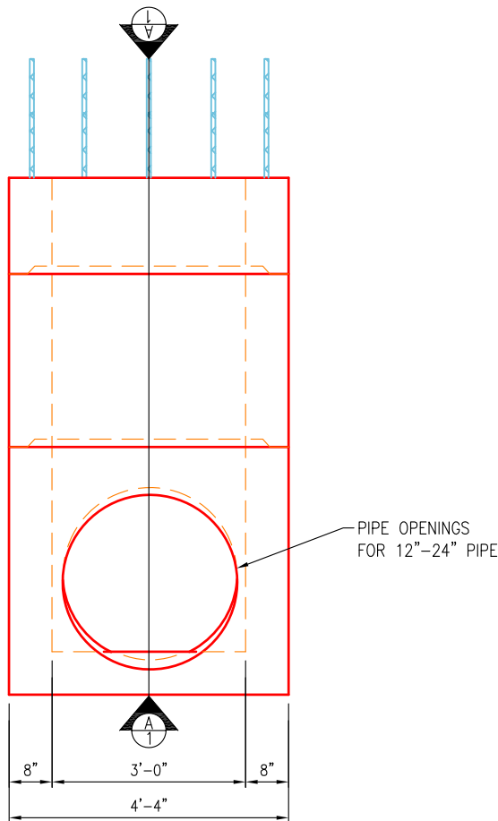
SIDE VIEW SCALE: 3/8" = 1'-0"
