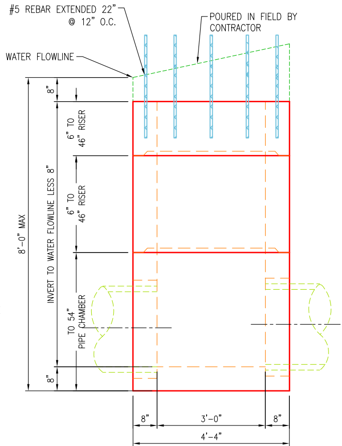
SECTION A-A SCALE: 3/8" = 1'-0"
