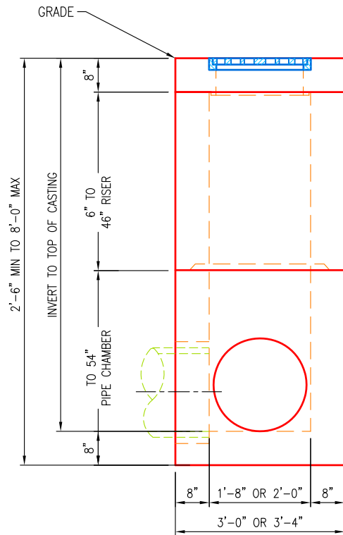
SECTION A-A SCALE: 3/8" = 1'-0"
