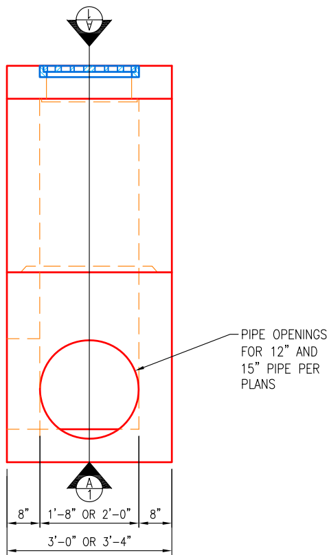
SIDE VIEW SCALE: 3/8" = 1'-0"
