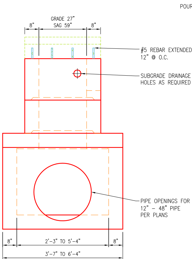
SIDE VIEW SCALE: 3/8" = 1'-0"
