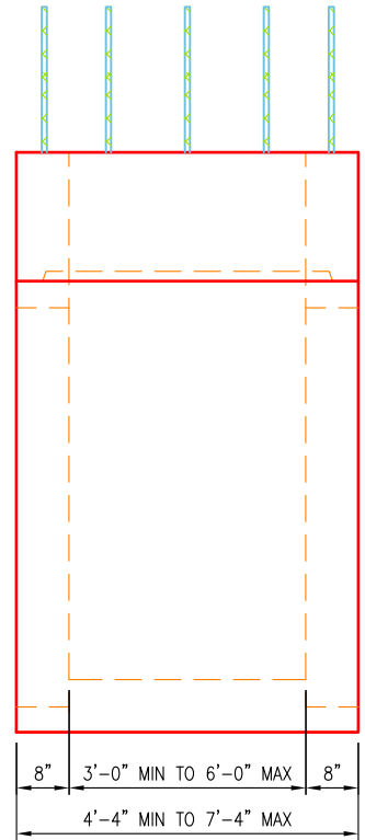
END VIEW SCALE: 3/8" = 1'-0"
