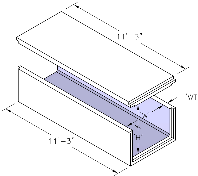
Trench Type-I Top
