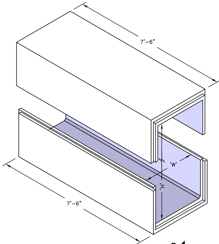
Trench Type-II Top
