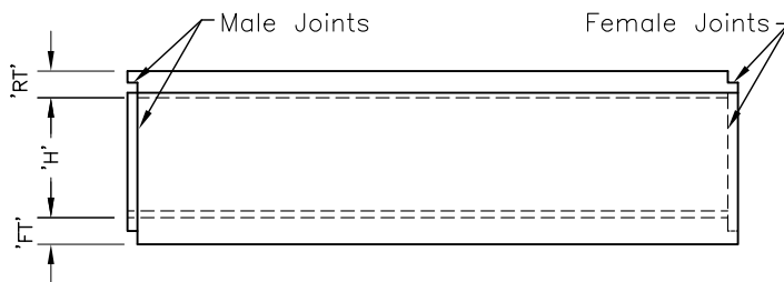
ELEVATION A-A
