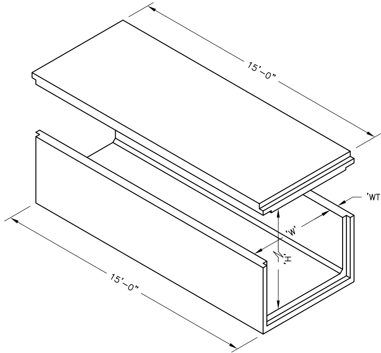
Box Culvert Type-I Top
