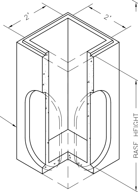
2'x2' BASE
