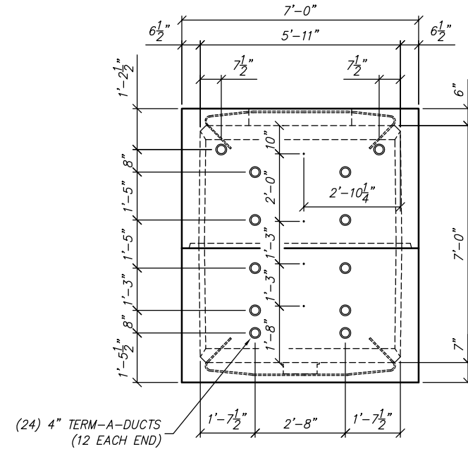
END VIEW SCALE: 1/4" = 1'-0"
