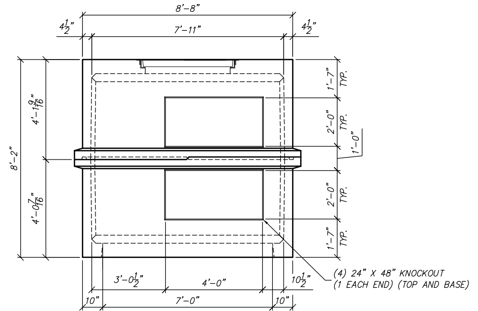
END VIEW SCALE: 1/4" = 1'-0"
