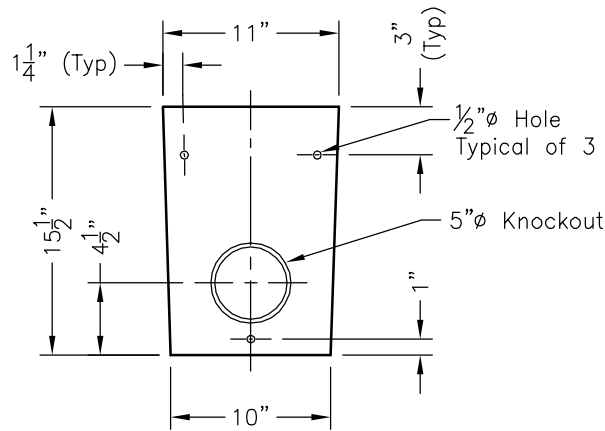
ELEVATION C-C
