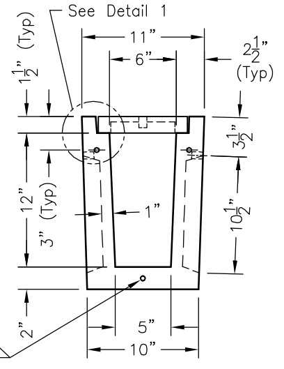
ELEVATION B-B
