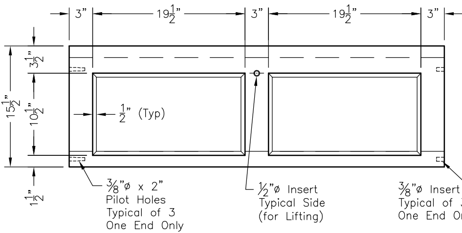
ELEVATION A-A
